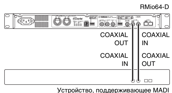
Устройство, поддерживающее MADI
