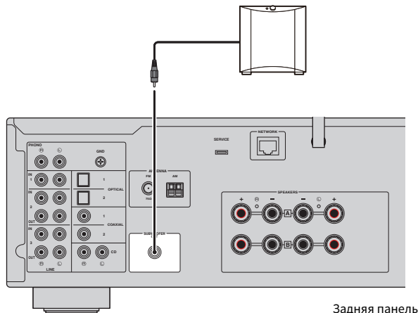
Задняя панель
