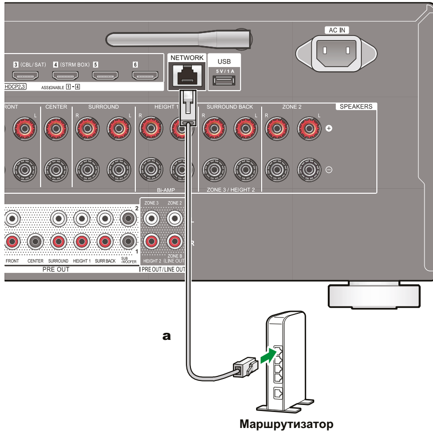
a Ethernet-кабель
