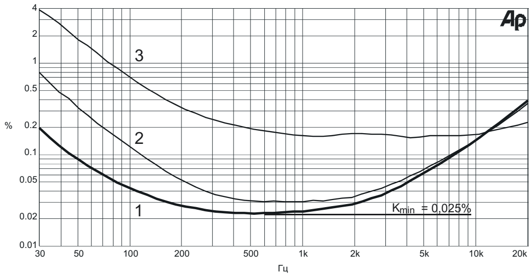
График зависимости коэффициента искажений (в %) от частоты при 3 Вт и 4 Ом от 30 Гц до 20 кГц при различных вариантах настройки тока покоя
