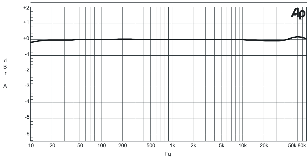
Частотная характеристика (10 Гц – 90 кГц, отклонение не более 0.3 дБ)
