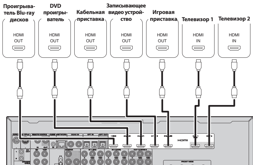
[Задняя панель]
