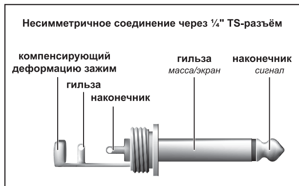
Рис. 6.2: 6,3-мм моноштекер
